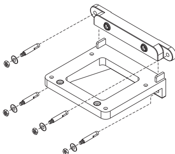
牆壁固定方式
